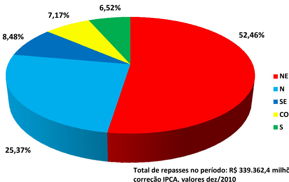
Fig. 6 – Distribuição regional dos recursos do FPE no período 2001 a 2010 – valor descontado de FUNDEF/FUNDEB.
