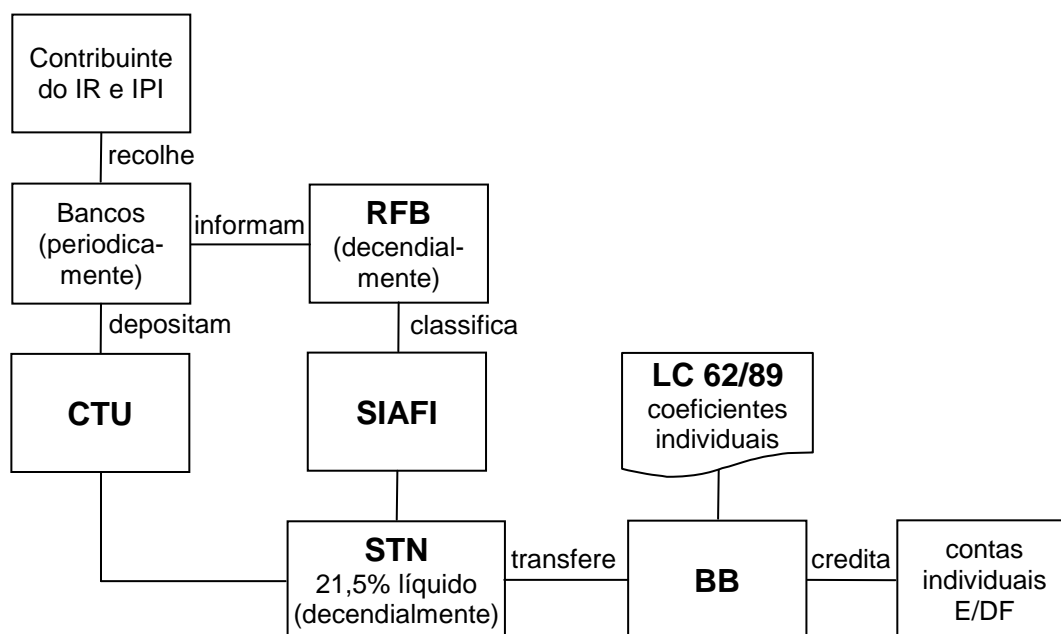
Fig. 3 – Fluxo de recursos das transferências do FPE.
