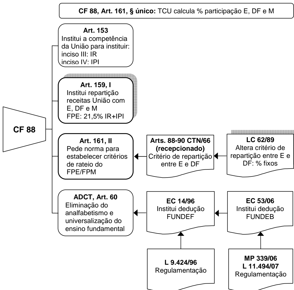
Fig. 2 – Inter-relação entre a legislação sobre transferências do FPE.
