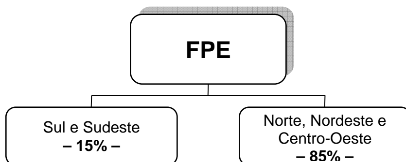
Fig. 4 – Distribuição regional do FPE.
