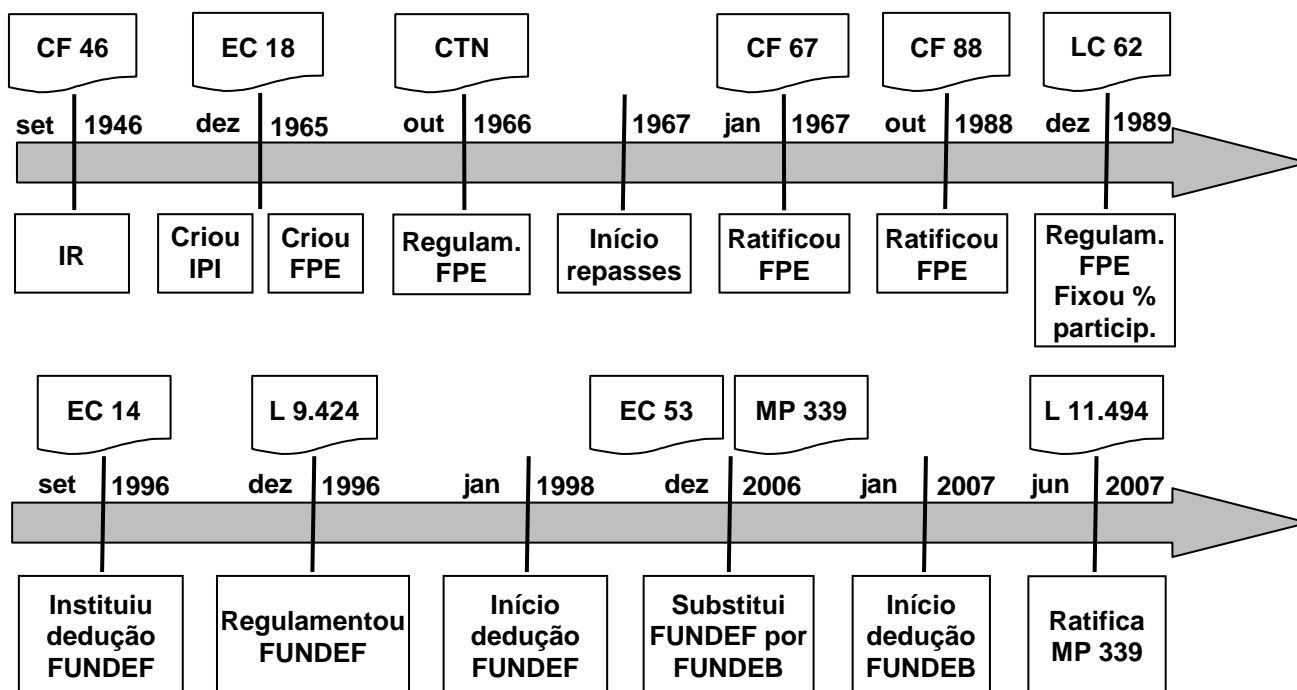
Fig. 1 – Histórico da legislação sobre FPE.
