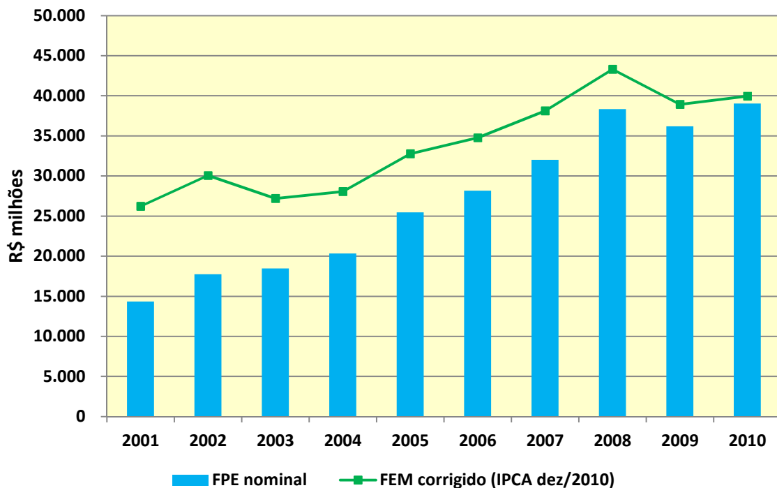
Fig. 5 – Evolução anual das transferências intergovernamentais do FPE – valores descontados de FUNDEF/FUNDEB.
